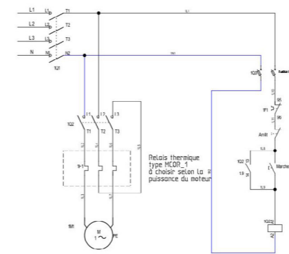
DÉMARRAGE DIRECT POUR MOTEUR MONOPHASE 230V PILOTAGE EN 230V
