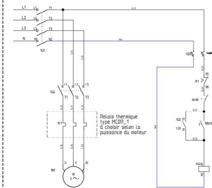
DÉMARRAGE DIRECT POUR MOTEUR TRIPHASE 400V PILOTAGE EN 230V
